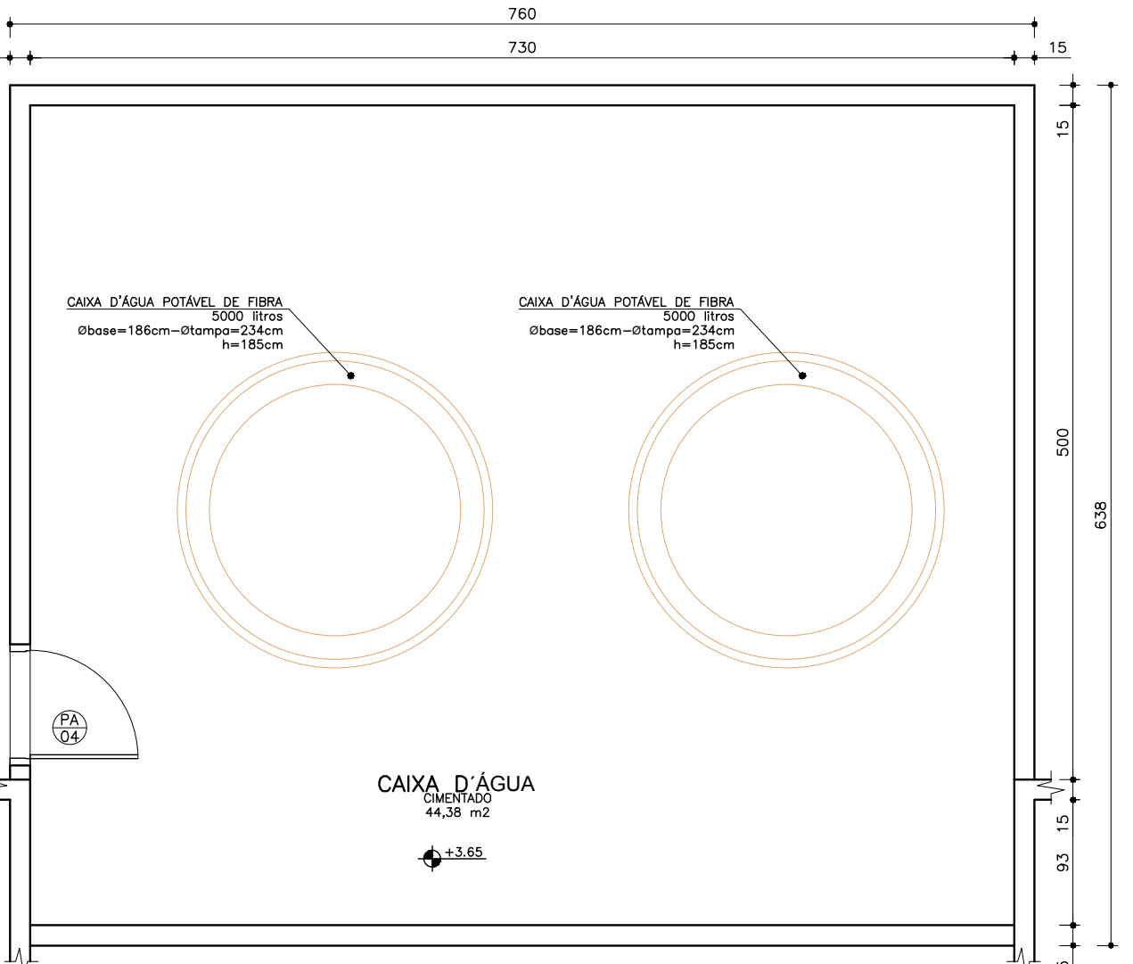
Planta Baixa Caixa D'água Esc: 1:50
