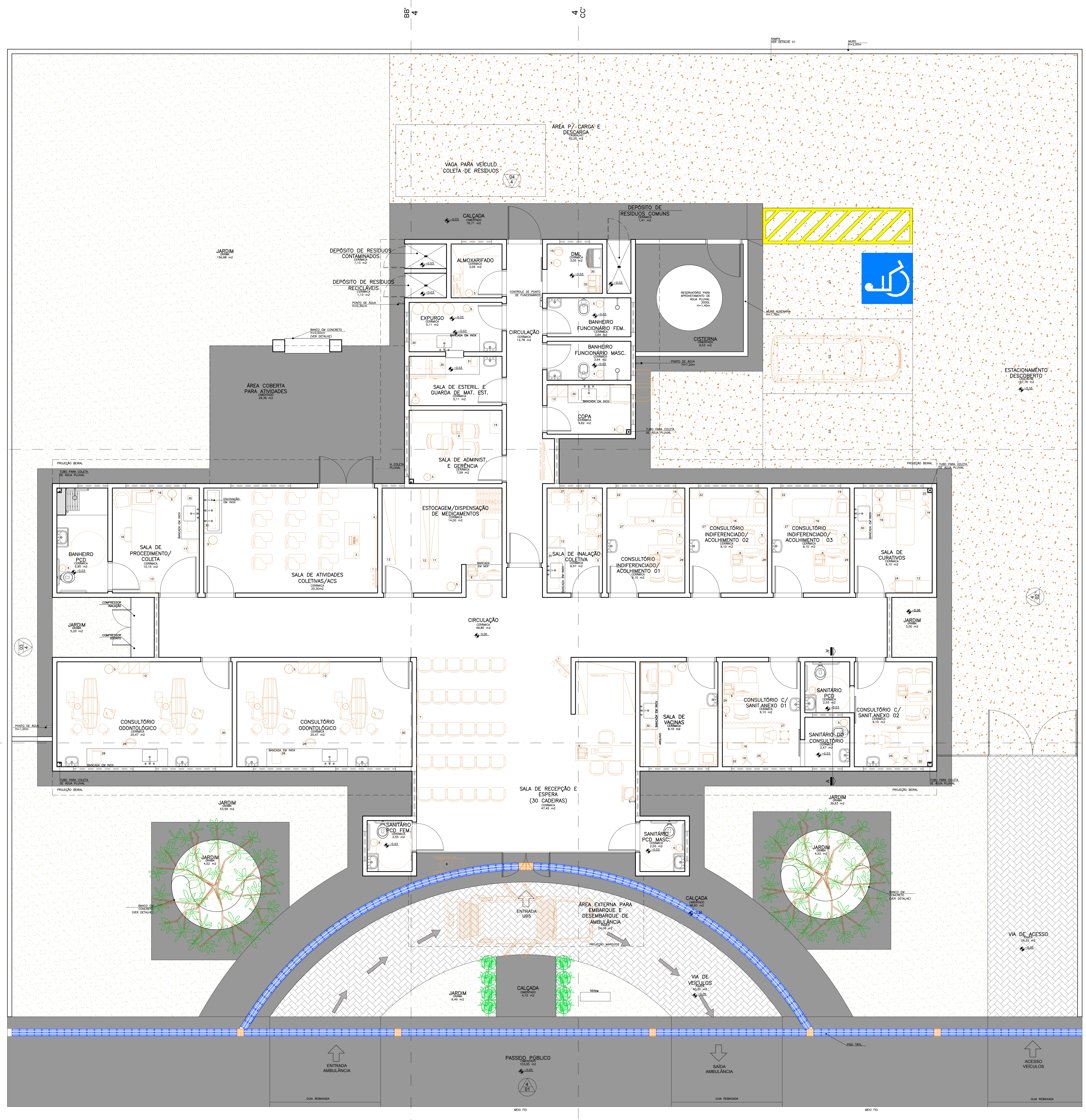
Planta Baixa Layout Nível: 0,00m Escala: 1:150 Área: 385,57m 2
