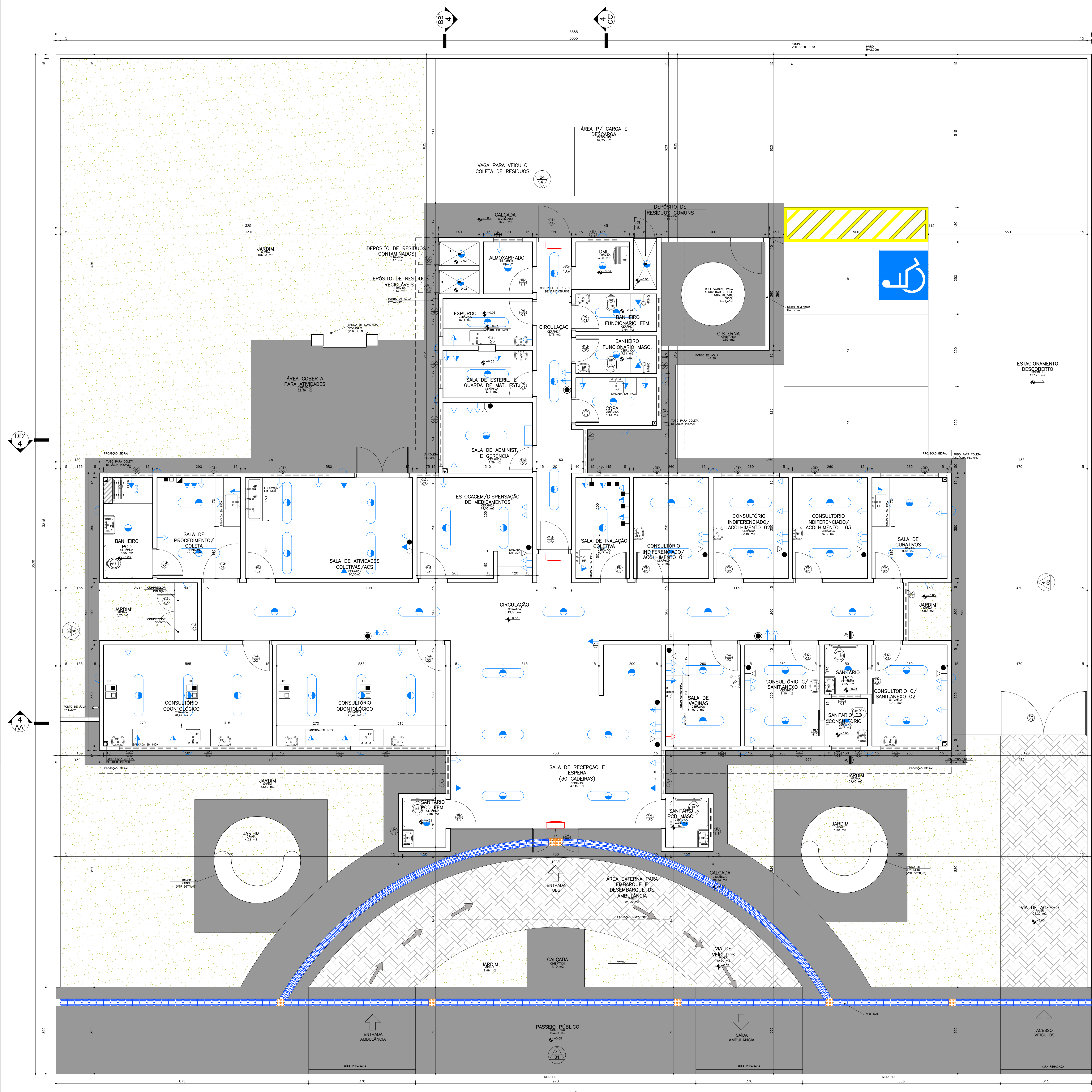
Planta Baixa e Instalações Nivel: 0,00m Esc.: 1:50 Área: 385,57m²
